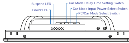
Right I/O
