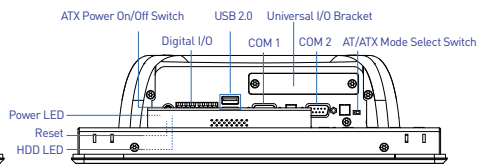
Right I/O
