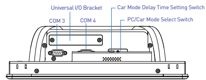
Right I/O
