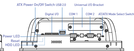
Right I/O
