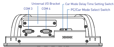
Right I/O
