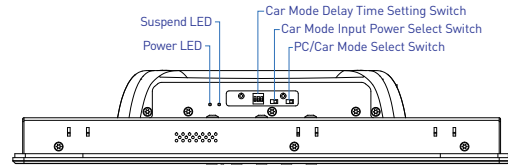
Right I/O
